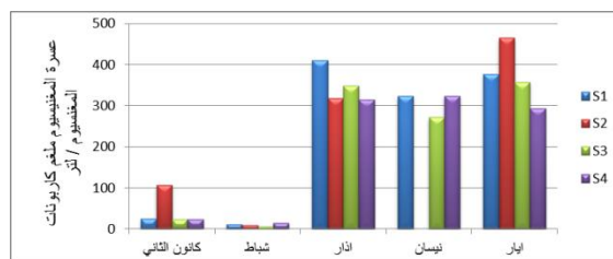
الشكل (11): بوضوح التغيرات الشهرية والموقعية لعسرة المغنيسيوم (ملغم كاربونات المغنيسيوم/ لتر) في وحدة المعالجة خلال عام 2014
