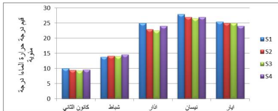
الشكل(2): يوضح التغيرات الشهرية و الموقعية لدرجة حرارة الماء (درجة مئوية) في وحدة المعالجة خلال عام 2014
