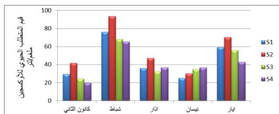
الشكل (7): يوضح التغيرات الشهرية والموقعية للمتطلب الحيوي للأوكسجين (ملغم / لتر) في وحدة المعالجة خلال عام 2014
