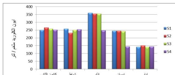
الشكل (12): بوضوح التغيرات الشهرية والموقعية لتركيز ايون الكلوريد (ملغم / لتر) في وحدة معالجة خلال عام 2014
