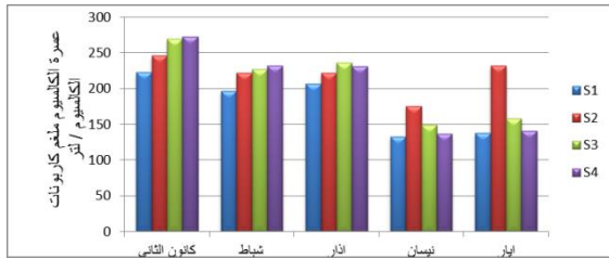
الشكل (10): يوضح التغيرات الشهرية والموقعية لعسرة الكالسيوم (ملغم كاربونات الكالسيوم / لتر) في وحدة المعالجة خلال عام 2014
